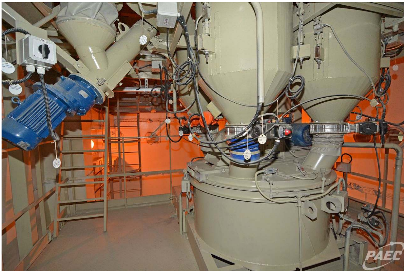
Роторний змішувач установки цементування з вузлом дозування
