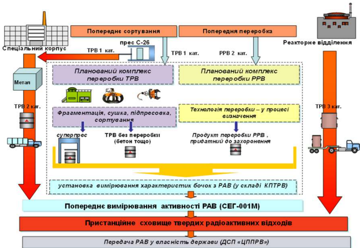
Перспективна схема системи поводження з ТРВ у ВП ЮУАЕС
