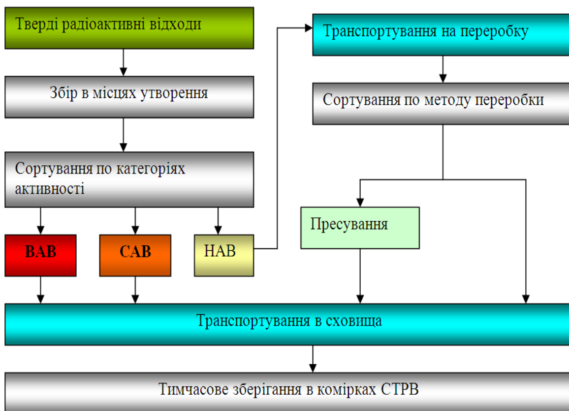
Схема поводження з ТРВ на ЮУАЕС
