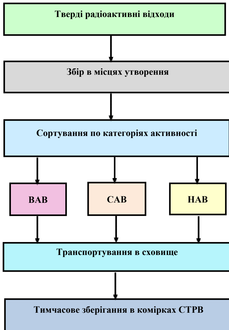
Схема поводження з ТРВ у ВП ХАЕС
