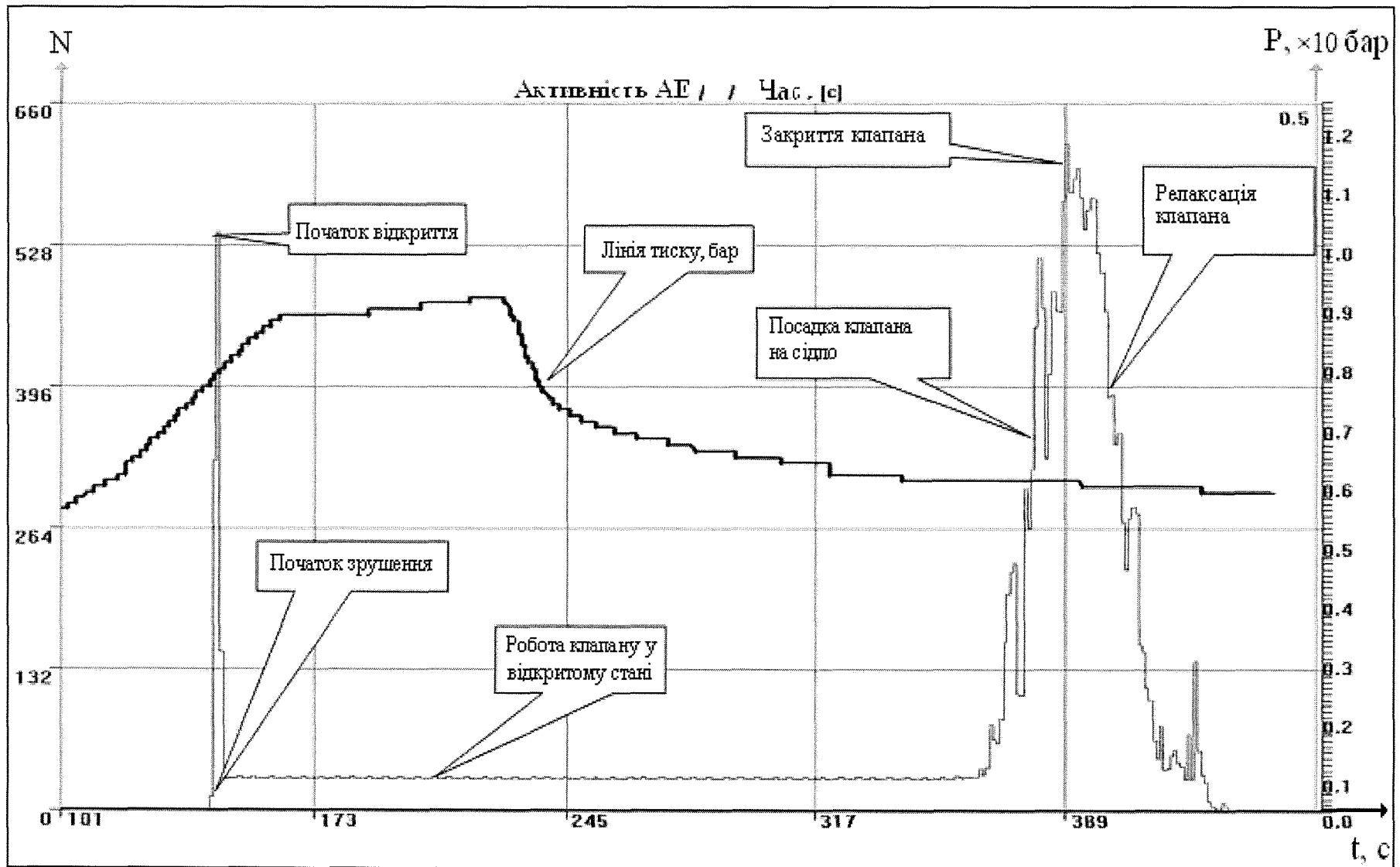
Рисунок 6.5.1 - Графік ідентифікації робочих процесів у запобіжному клапані за сигналами АЕ
